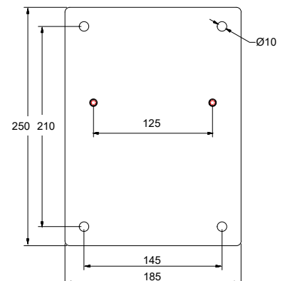
Avlastningsplåt för stålfasader eller andra svaga fasader.
